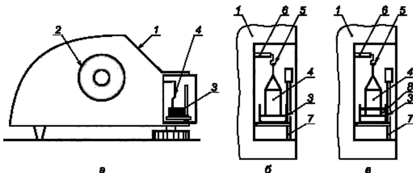
а — общий вид; б, в — фрагменты измерительной части; 1 — торсионные весы; 2 — ручка измерительного барабана; 3 — измерительная ювета с жидкостью; 4 — кольцо; 5 — крючок для подвешивания измерительного кольца; 6 — коромысло измерителя; 7 — штатив; 8 — горячая жидкость
